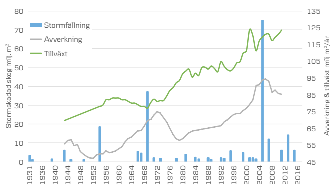
Figur 3. Sammanställning av dokumenterade stormskador på skog > 1 miljon m 3 per år under 100 år.
