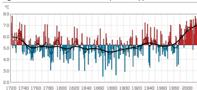
Figur 1. Rekonstruerad årsmedeltemperatur, Uppsala 1722–2018
